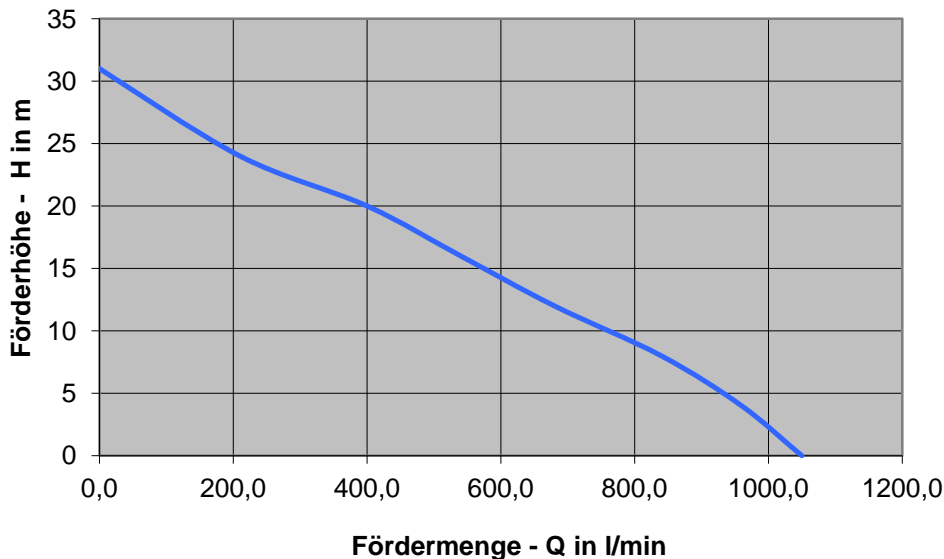
Kennlinie - Diesel-Motorpumpe HL80CLE
