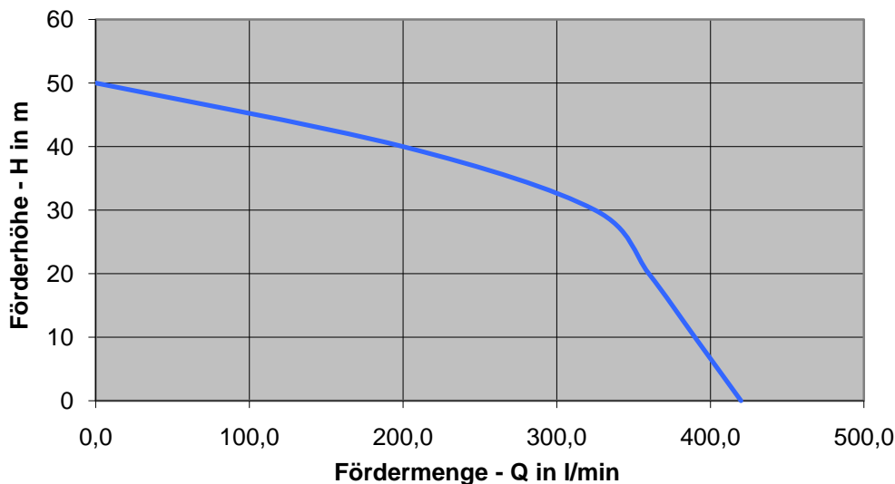
Kennlinie - Dieselmotorpumpe HL50CXLE
