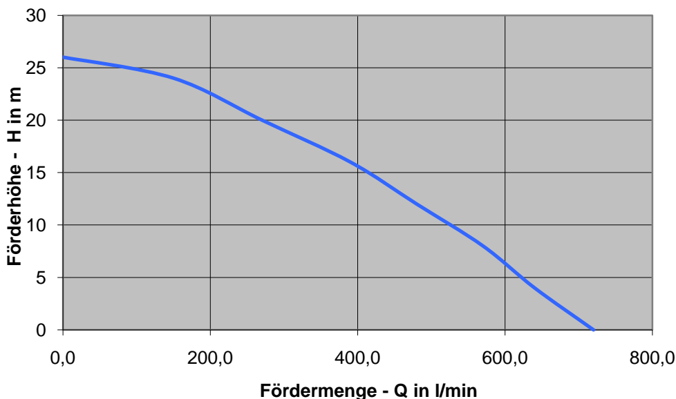
Kennlinie - Diesel-Motorpumpe HL50CLA
