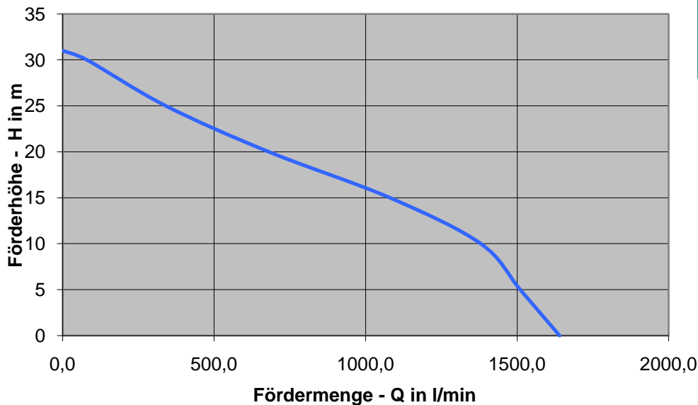
Kennlinie - Dieselmotorpumpe HL100CLE
